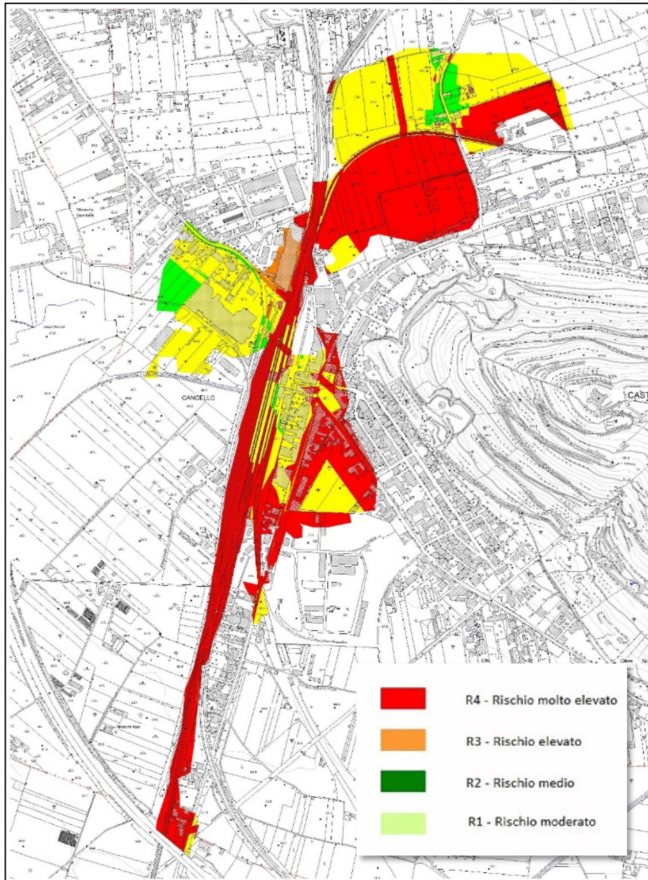
Comune di San Felice a Cancellò (CE) lago Carmignano - Piano Stralcio di Assetto idrogeologico dell'ex AdB Campania Centrale - Stralcio mappa del Rischio idraulico approvato - tavv. 431143Ri, 448011Ri.
