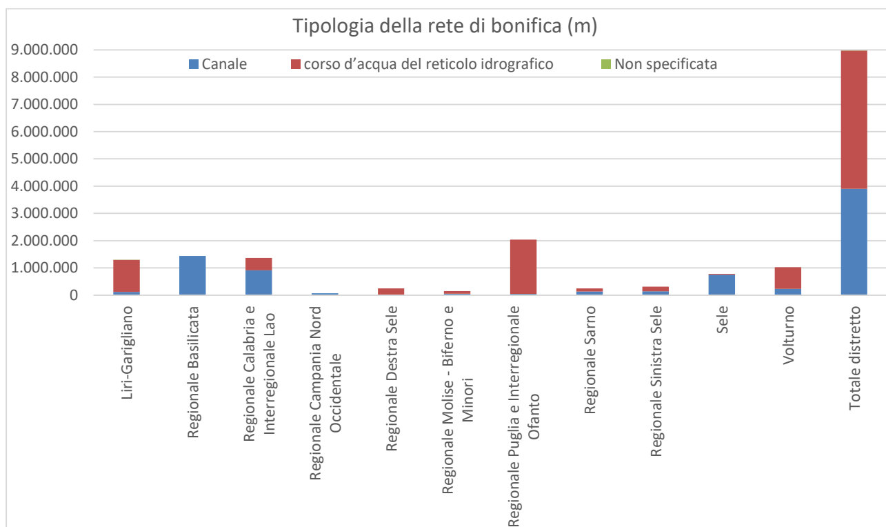
Figura 16. Tipologia delle reti di bonifica (dati per UoM) – FONTE Elaborazione CREA su dati dei Consorzi
