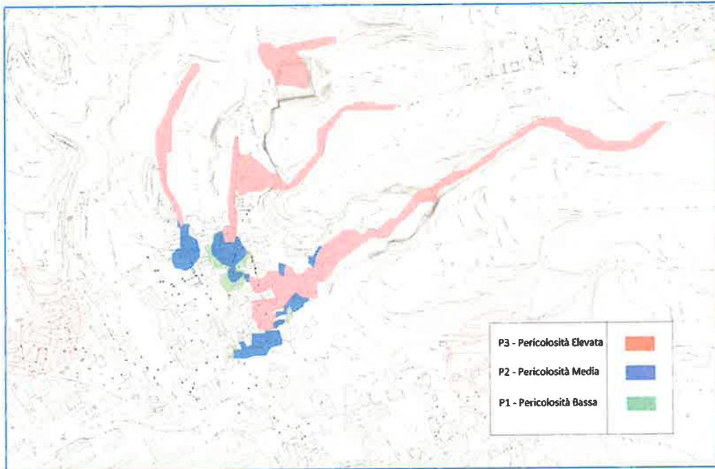
Comune di Napoli – loc. via Grottole n.5- Piano Stralcio di Assetto idrogeologico dell'ex AdB Campania Centrale – Stralcio mappa della pericolosità idraulica proposta (tav. 477112P)
